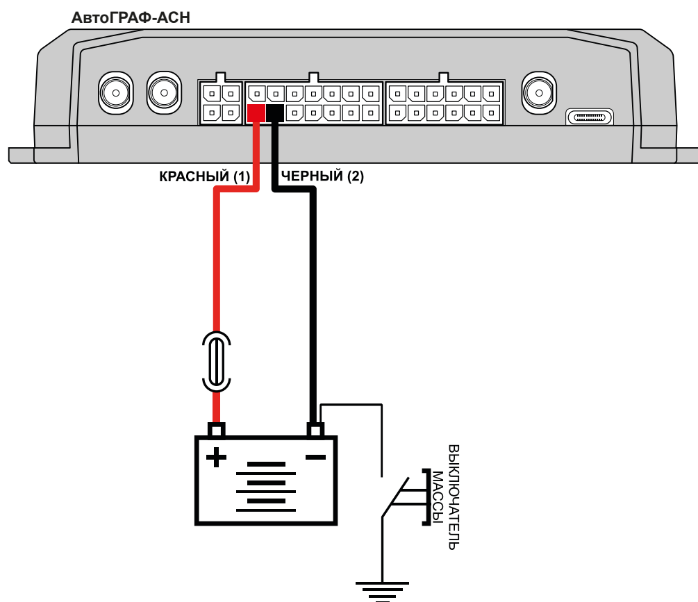
Рис.8. Подключение питания до выключателя массы
