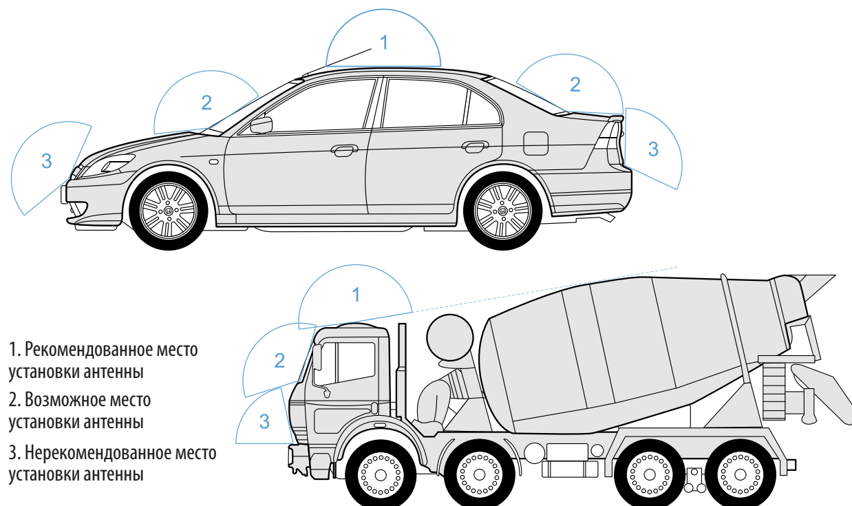
Рис.7. Установка ГЛОНАСС/GPS антенны
