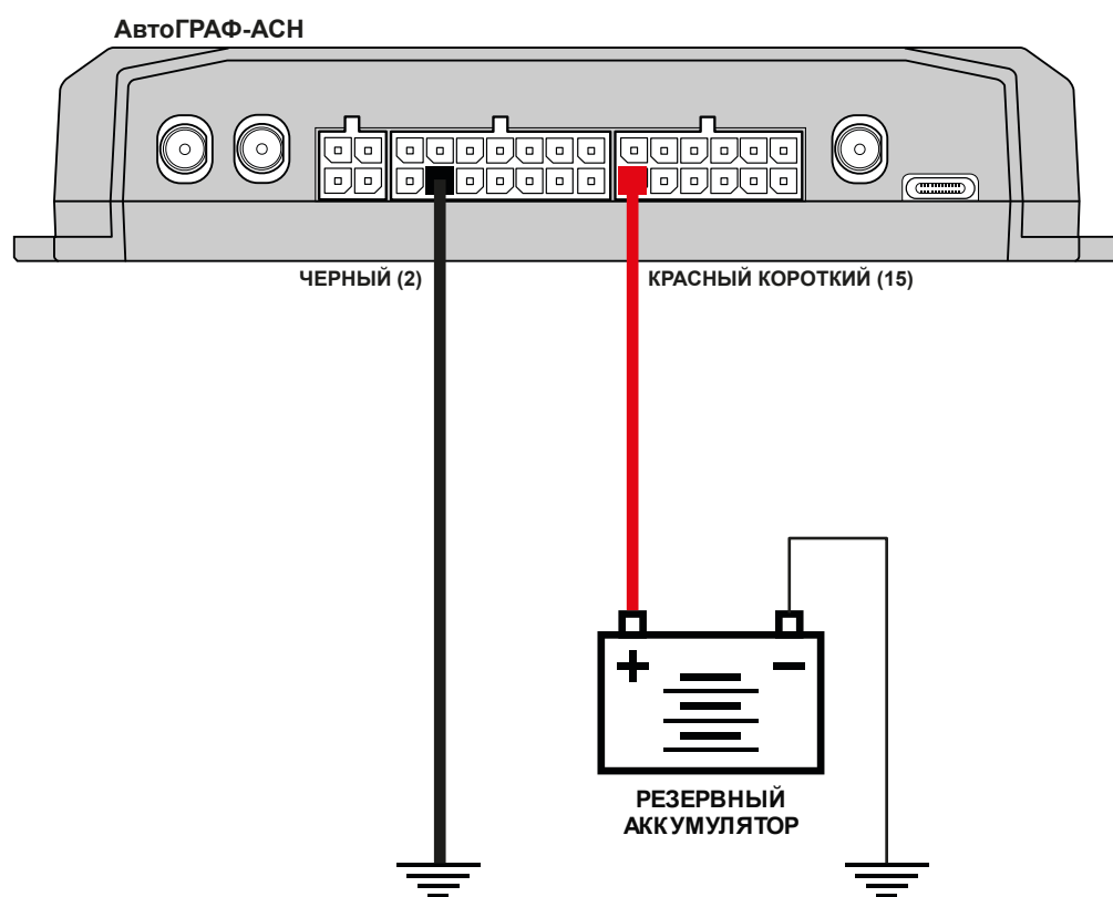
Рис.12. Установка резервного аккумулятора
