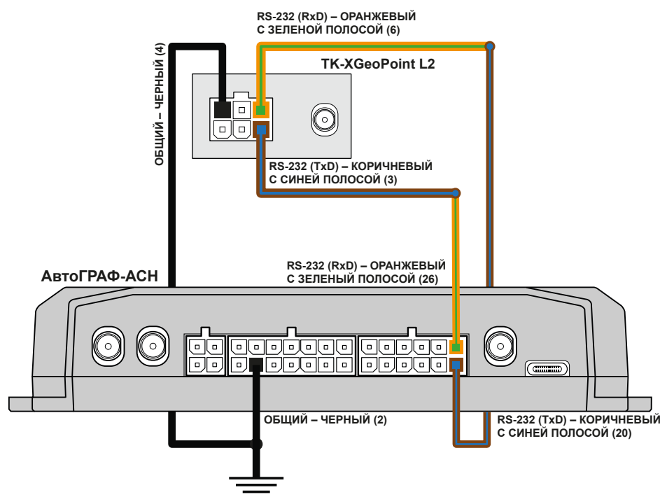
Рис.21. Схема подключения по шине RS-232
