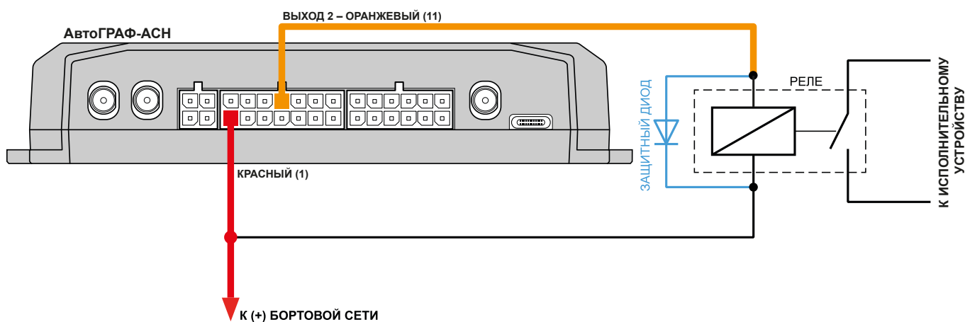
Рис.19. Схема подключения выхода
