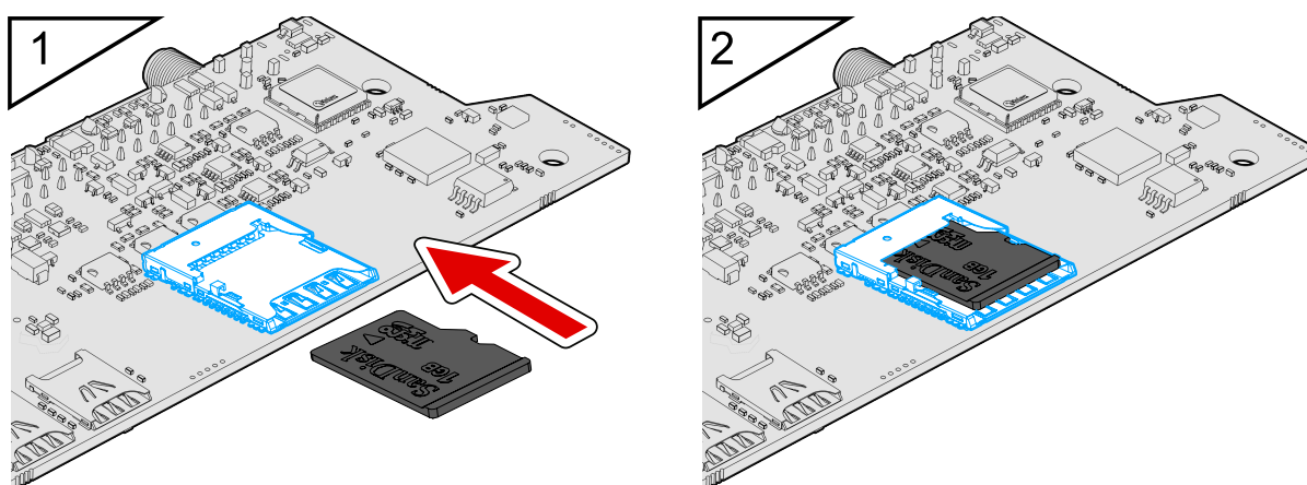
Рис.11. Установка SD-карты
