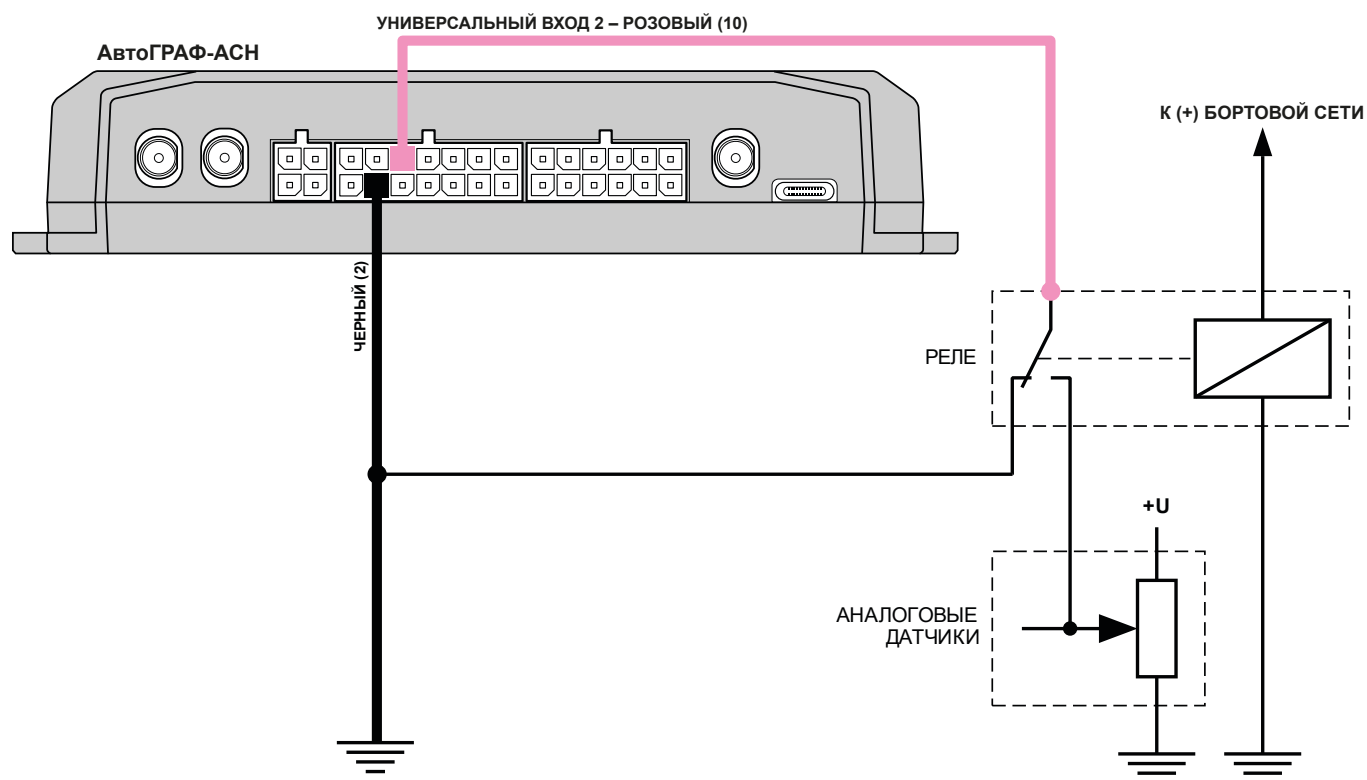
Рис.17. Подключение аналоговых датчиков к универсальному входу (схема с защитой от разрыва «массы»)
