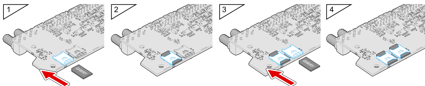
Рис.6. Установка SIM-карты пользователя
