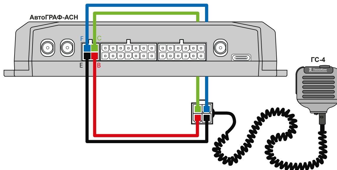
Рис.24. Схема подключения устройства громкой связи ГС-4
