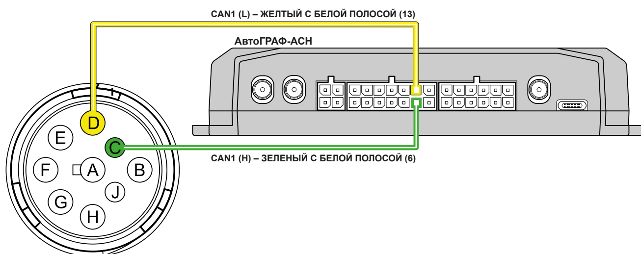
Рис.22. Схема подключения к шине CAN
