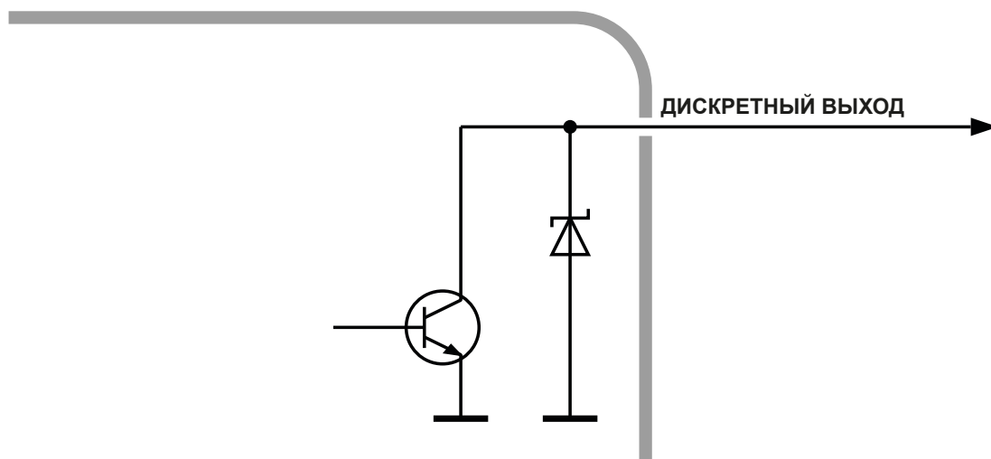
Рис.18. Внутренняя схема выхода
