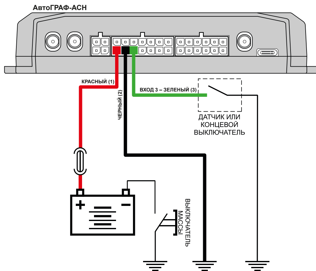
Рис.14. Подключение датчиков типа «сухой контакт» к универсальному входу
