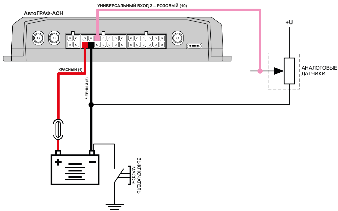
Рис.16. Подключение аналоговых датчиков к универсальному входу (схема без защиты от разрыва «массы»)
