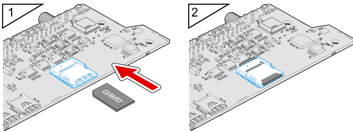
Рис.5. Установка SIM-карты оператора ГАИС «ЭРА-ГЛОНАСС»
