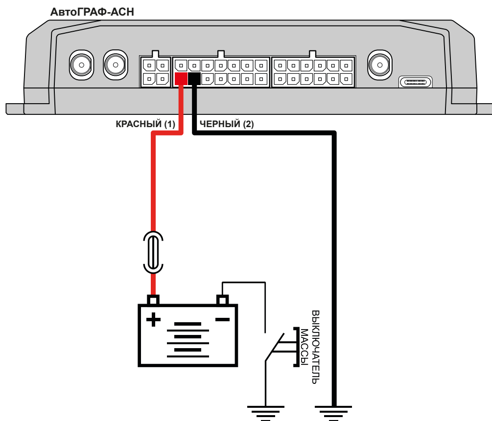
Рис.9. Подключение питания после выключателя массы
