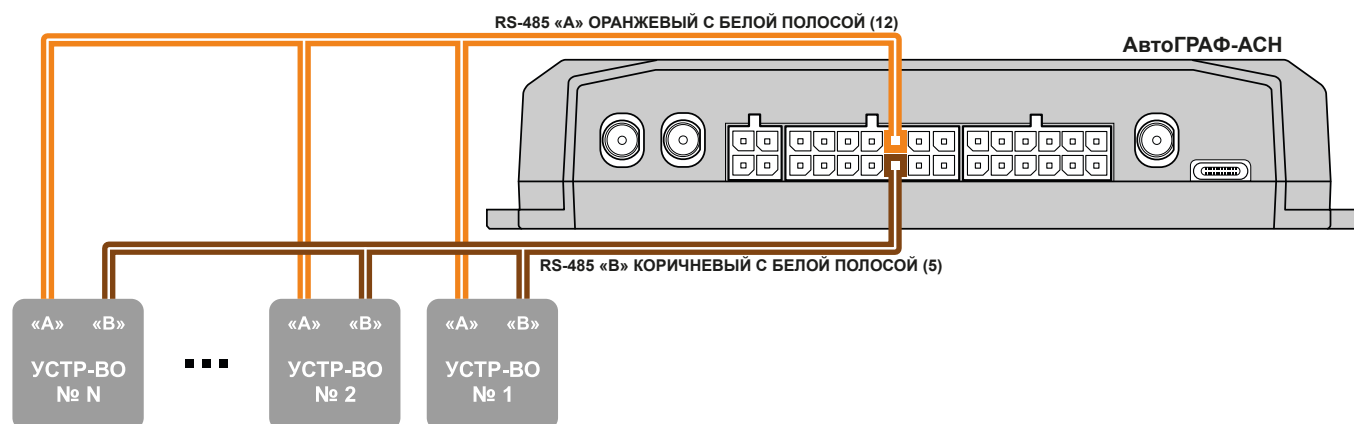
Рис.20. Схема подключения по шине RS-485
