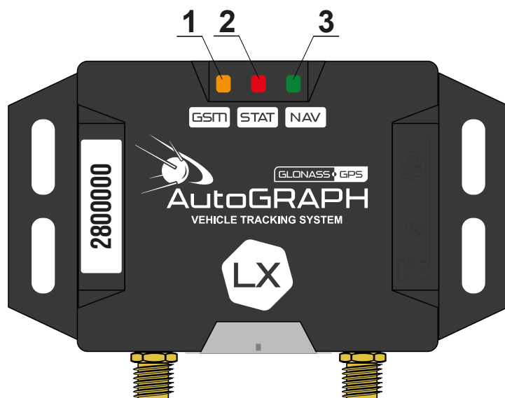
Рис.5. Индикация контроллера
