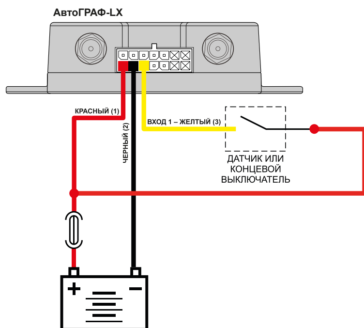
Рис.7. Подключение датчиков типа «сухой контакт» к универсальному входу
