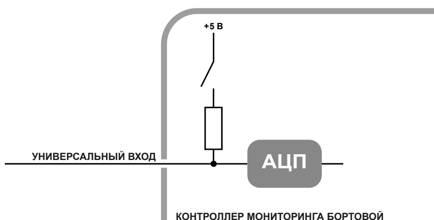
Рис.6. Внутренняя схема универсального входа
