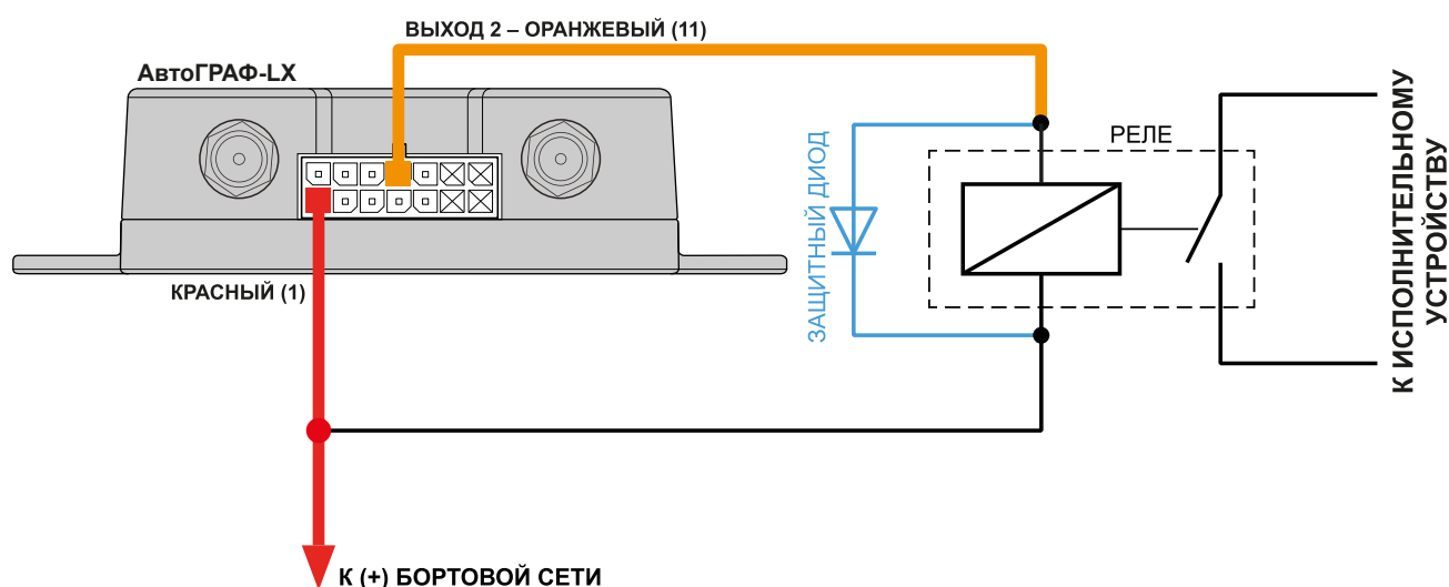
Рис.11. Схема подключения выхода
