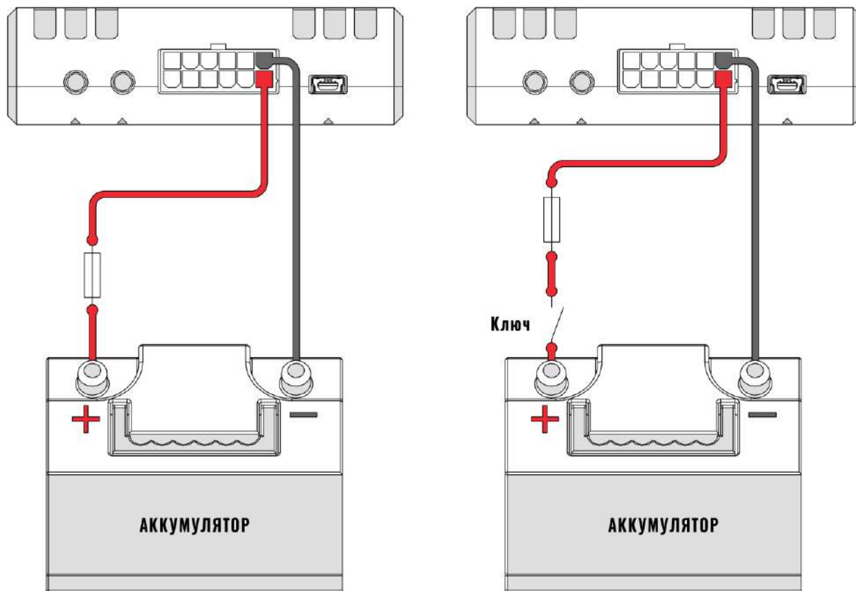
Рисунок 2.7 Подключение питания
