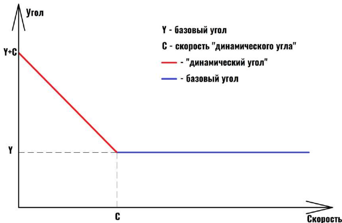
Рисунок 3.18 График зависимости динамического угла от скорости
