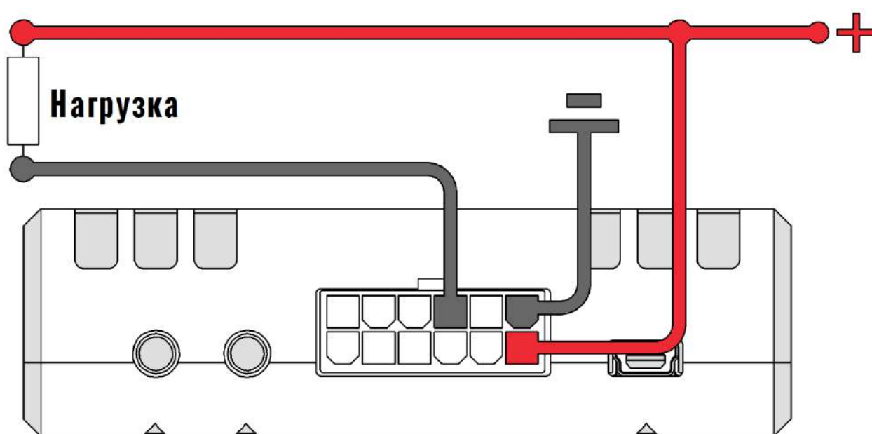
Рисунок 2.15 Подключение маломощной нагрузки
