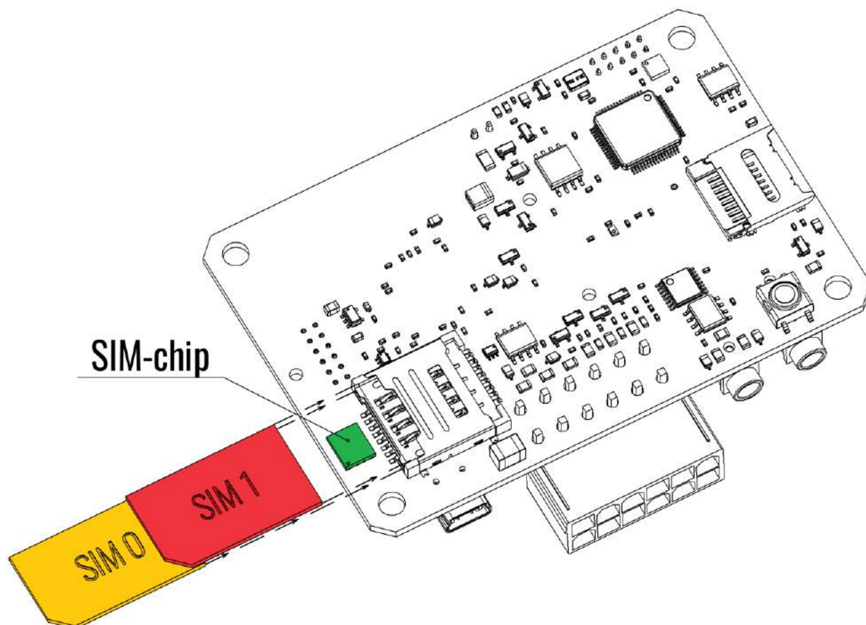
Рисунок 2.4 Установка SIM-карт
