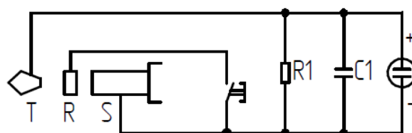
Рисунок 2.25 Схема распайки тангенты
