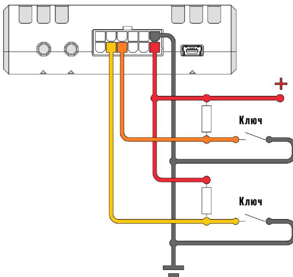
Рисунок 2.9 Подключение с подтяжкой к «+»
