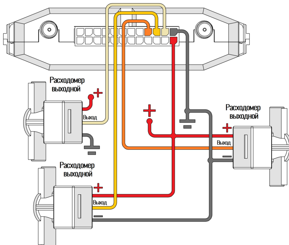
Рисунок 2.13 Пример подключения расходомеров в дифференциальном режиме
