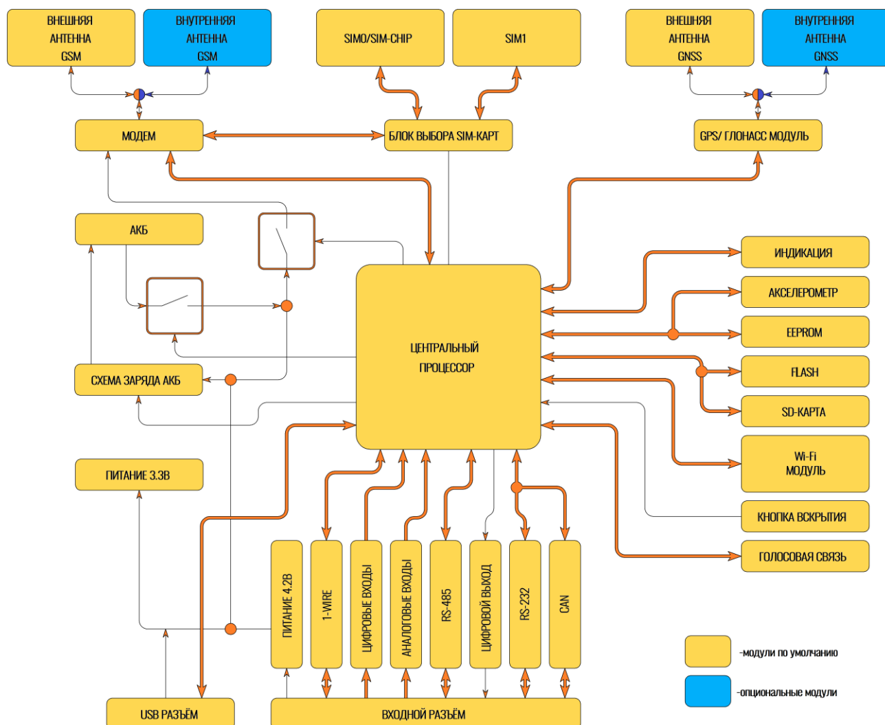
Рисунок 1.2 Блок-схема навигационного терминала
