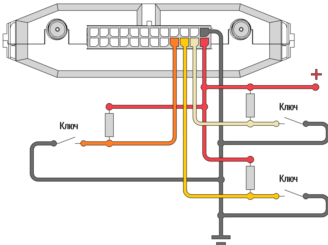
Рисунок 2.9 Подключение с подтяжкой к «+»
