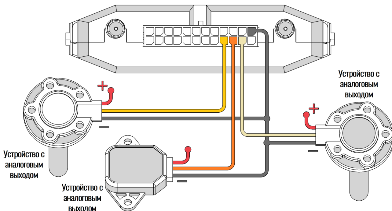
Рисунок 2.8 Подключение аналоговых источников
