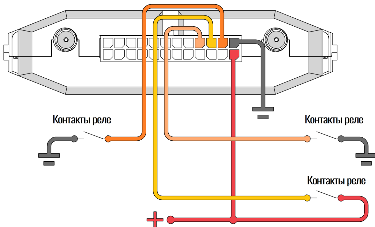
Рисунок 2.12 Варианты подключения дискретных датчиков
