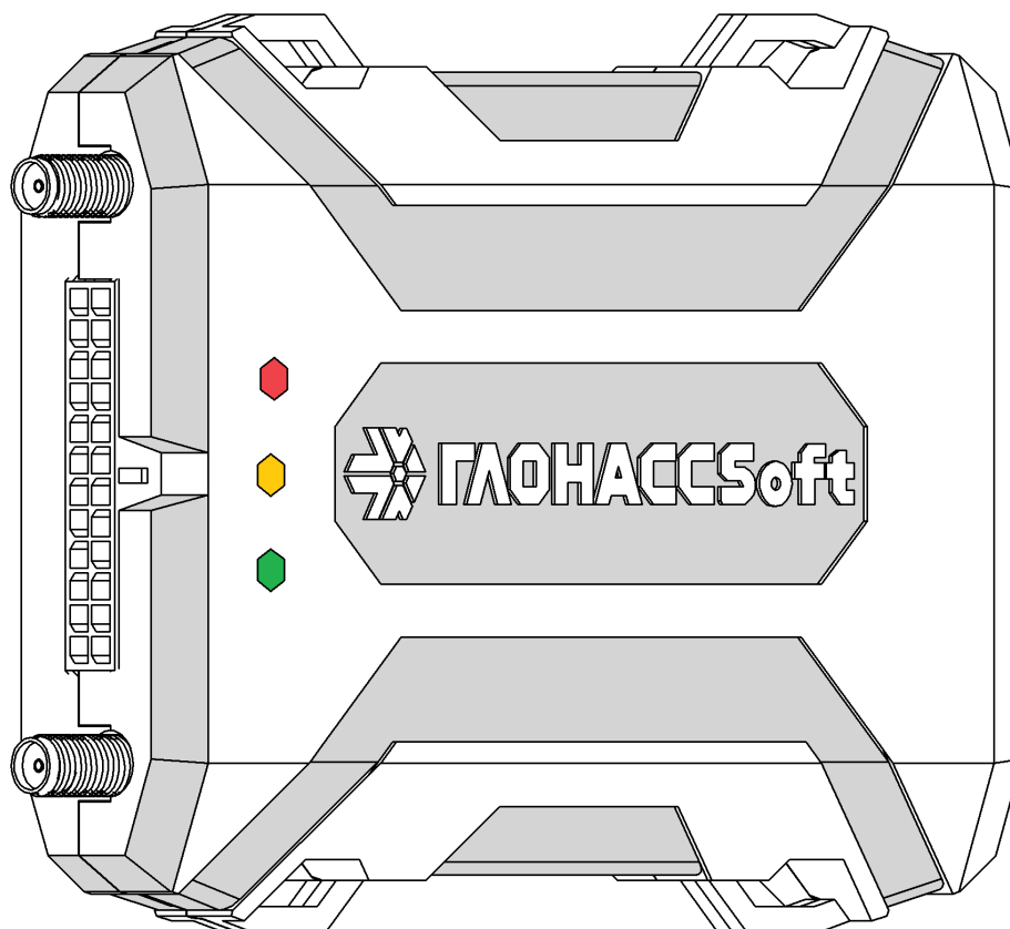
Рисунок 3.1 Расположение индицирующих светодиодов
