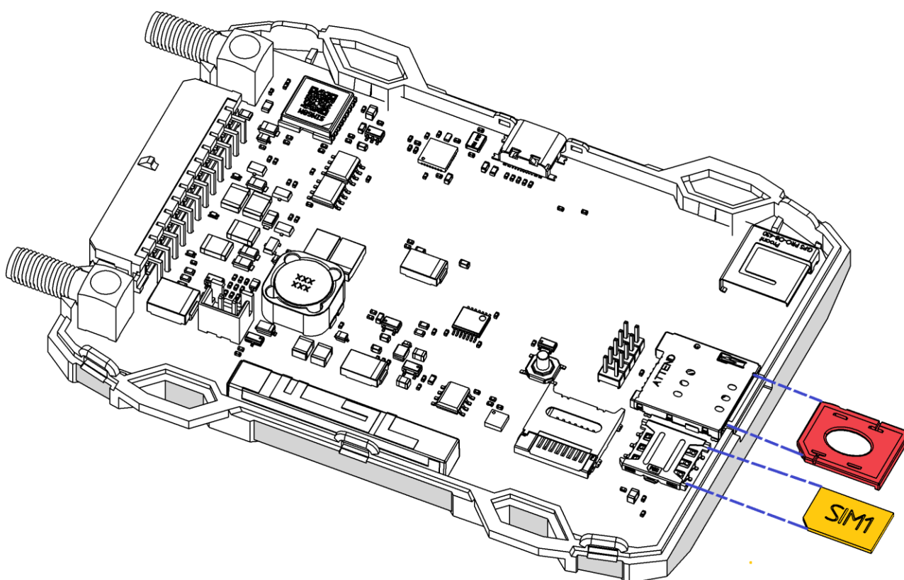
Рисунок 2.4 Установка SIM-карт
