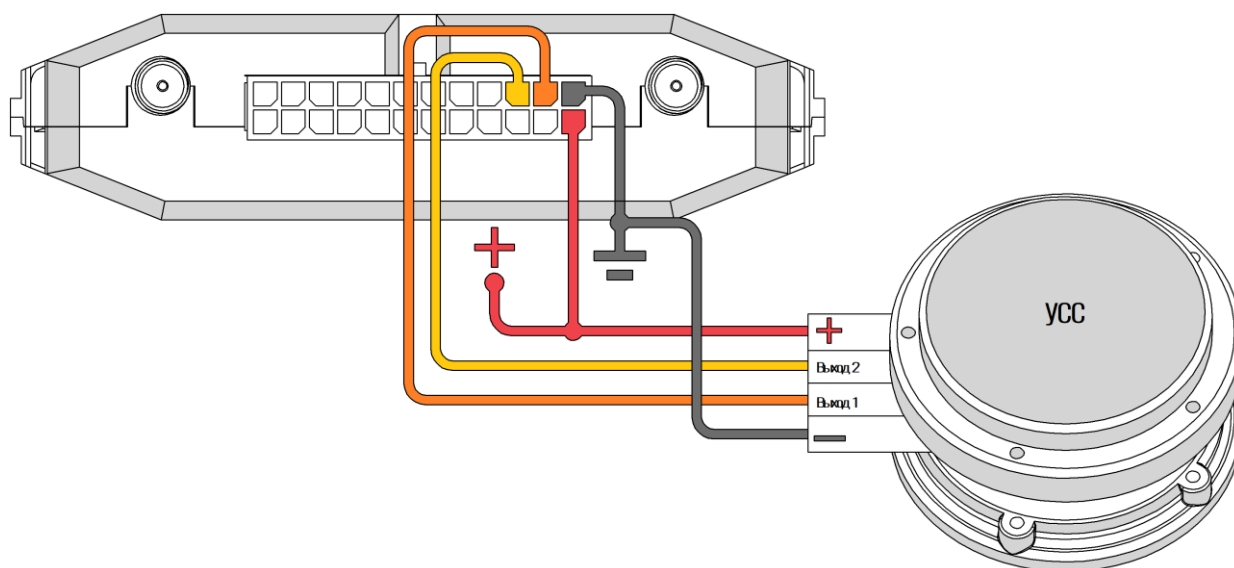
Рисунок 2.14 Пример подключения УСС
