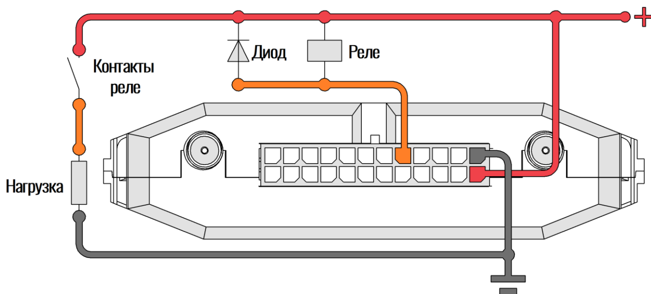
Рисунок 2.16 Подключение мощной нагрузки
