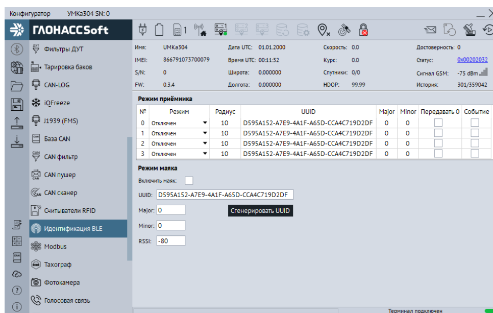
Рисунок 3.40 Вкладка «Идентификация BLE»
