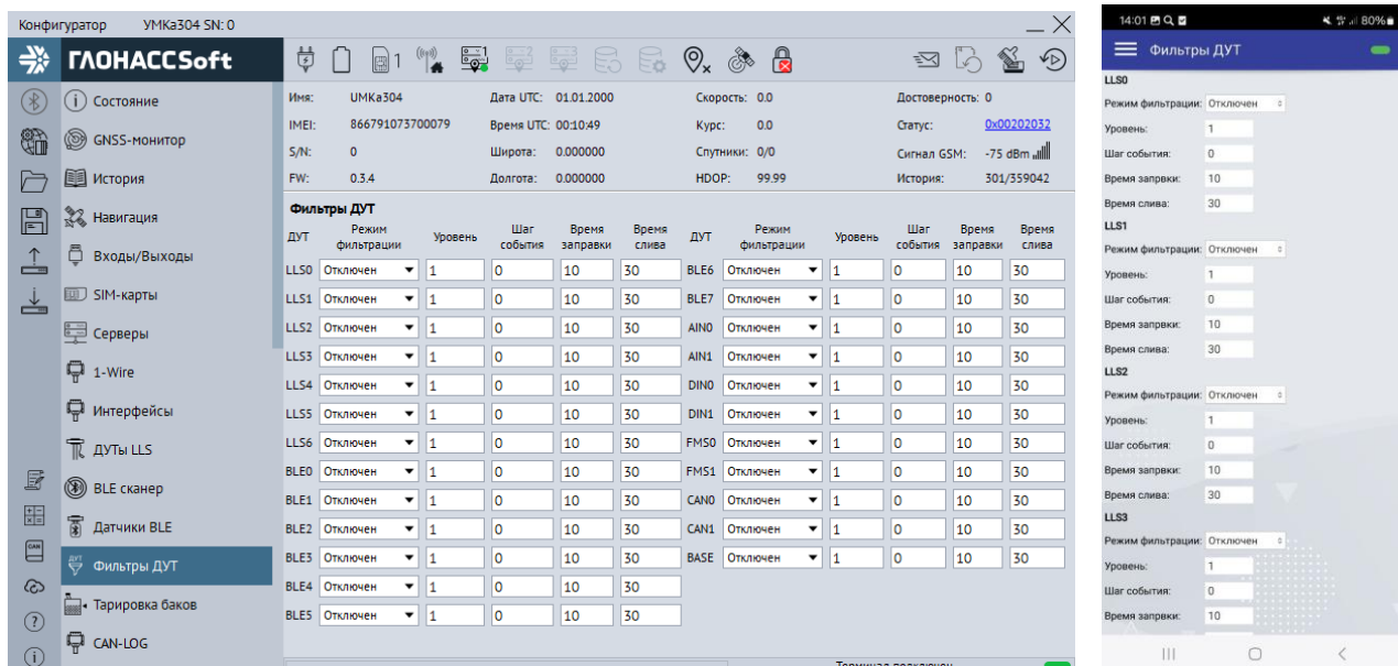
Рисунок 3.28 Вкладка «Фильтры ДУТ»
