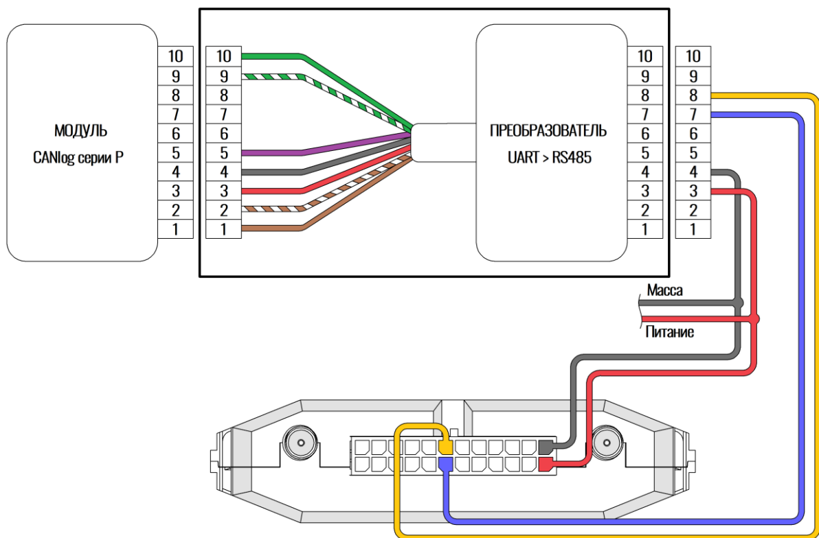
Рисунок 2.24 Подключение CAN-LOG через переходник UART-RS485
