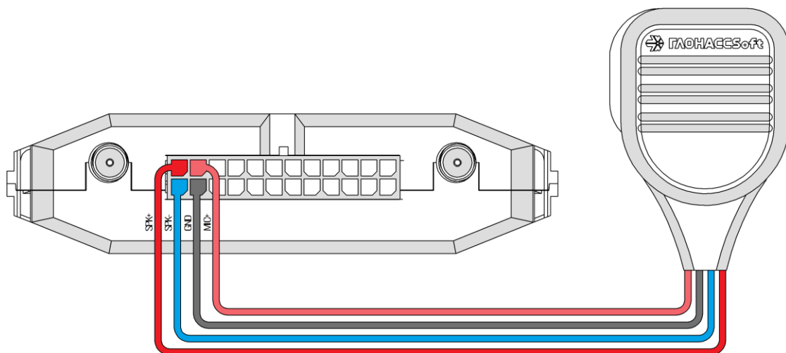
Рисунок 2.25 Схема подключения тангенты
