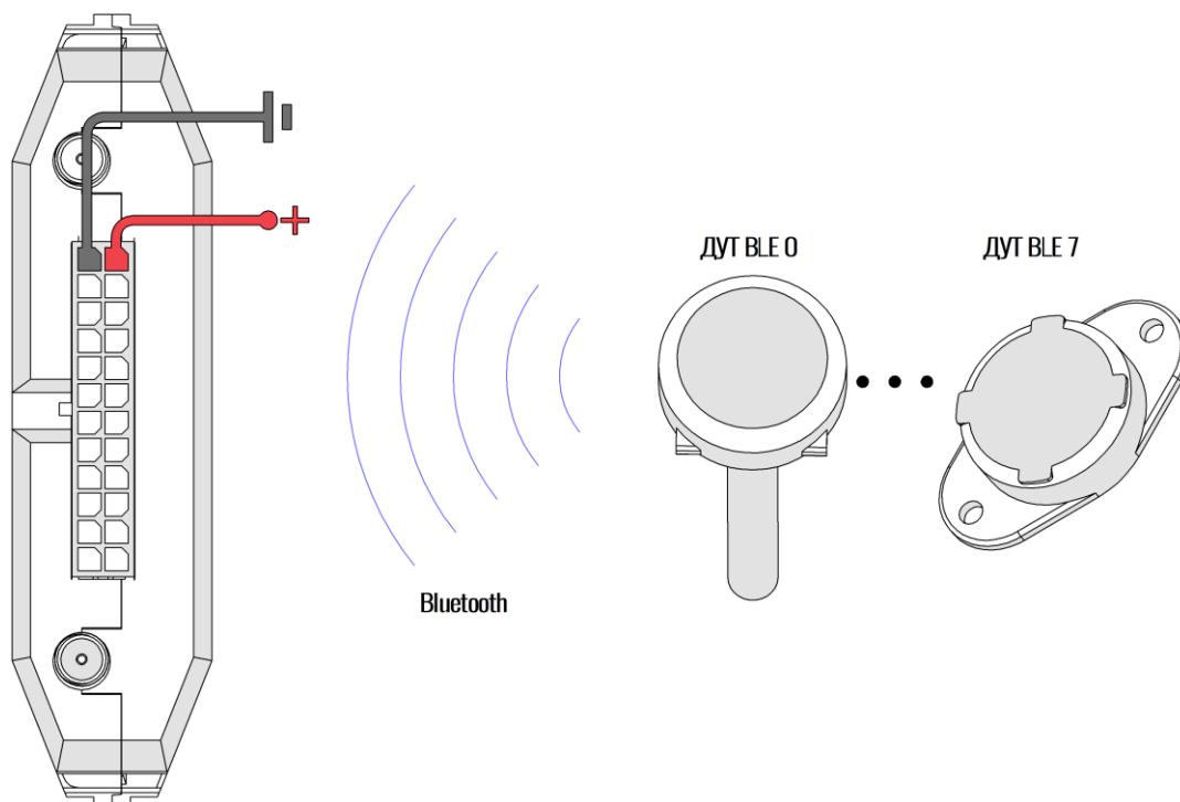
Рисунок 2.18 Подключение датчиков по BLE
