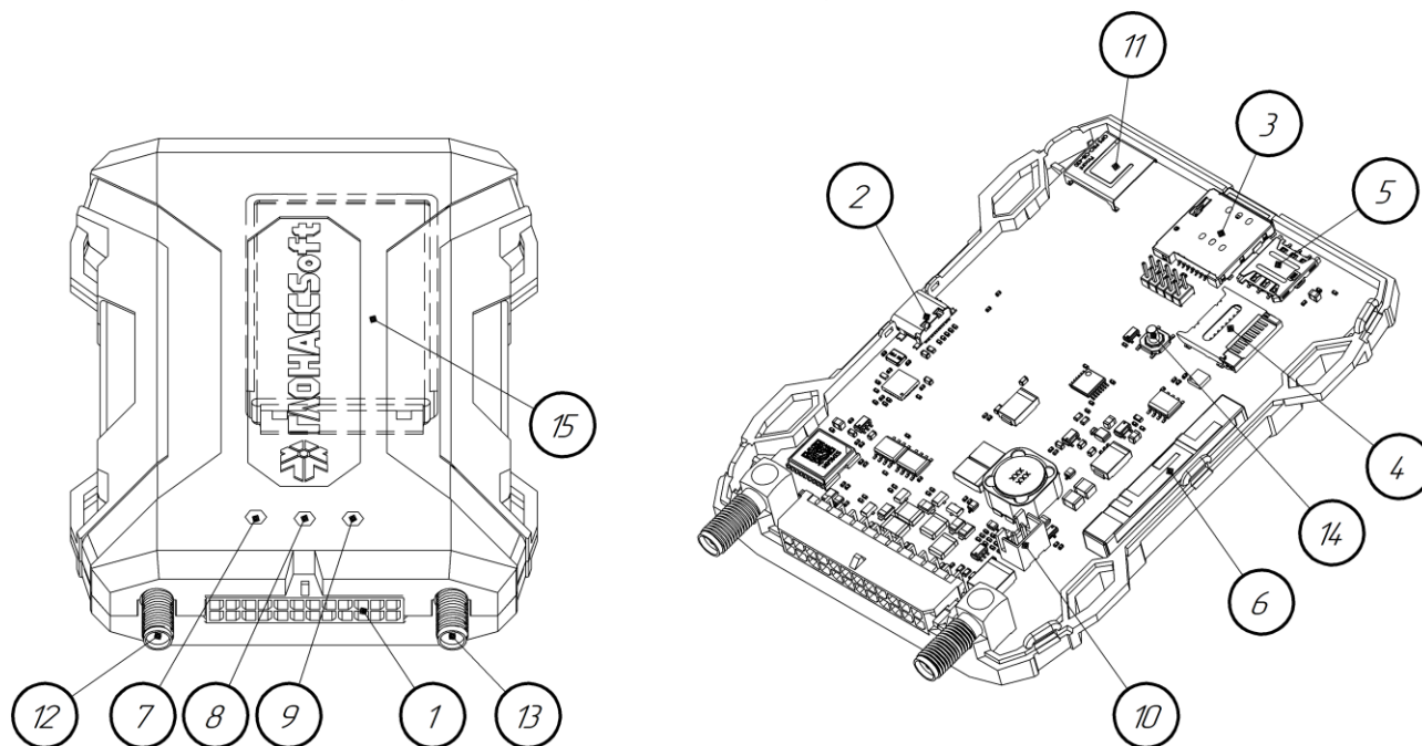
Рисунок 2.1 Основные элементы терминала
