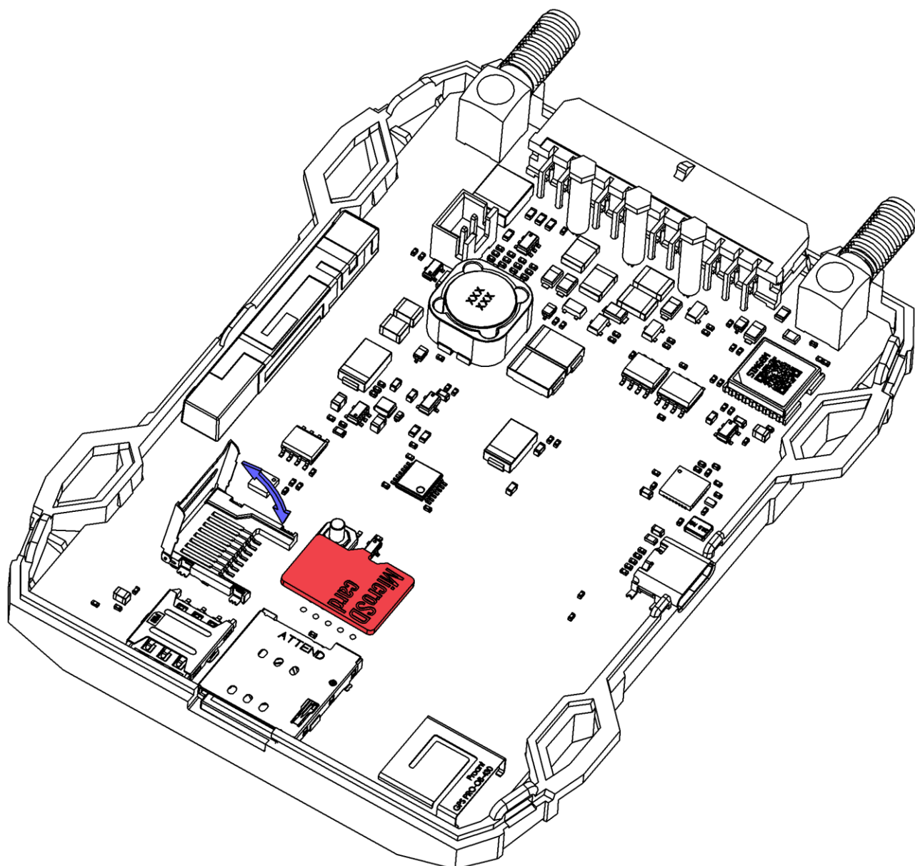
Рисунок 2.6 Установка microSD-карты
