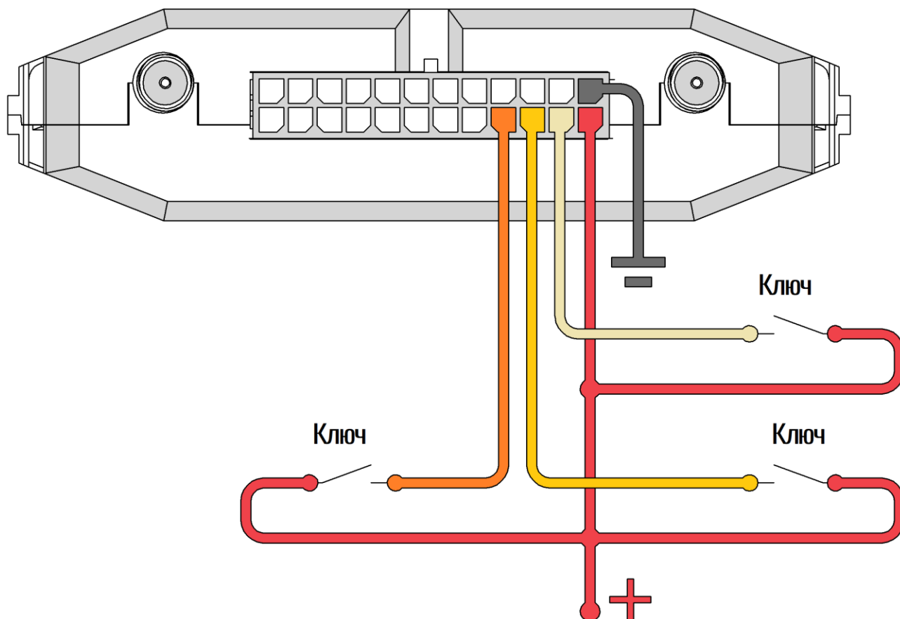
Рисунок 2.10 Подключение с подтяжкой к «-»
