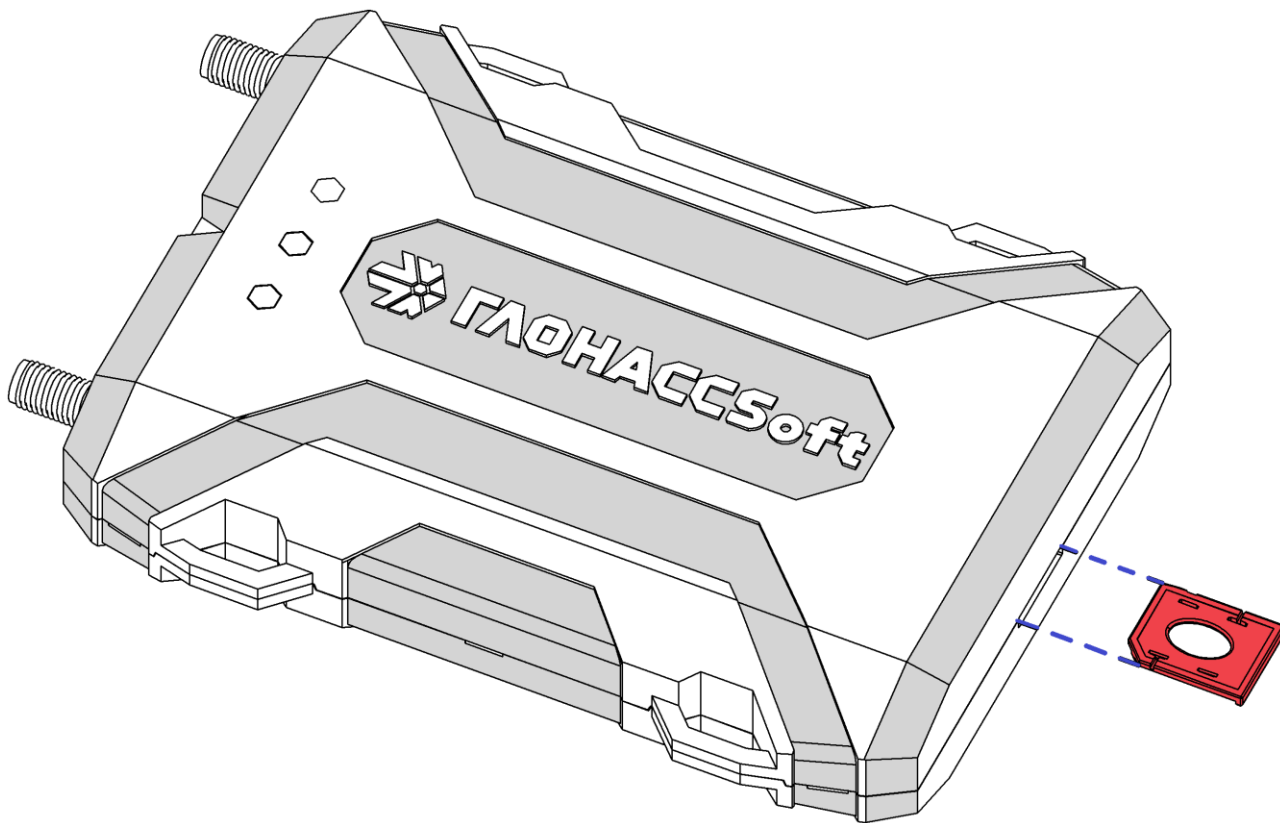
Рисунок 2.3 Установка SIM0
