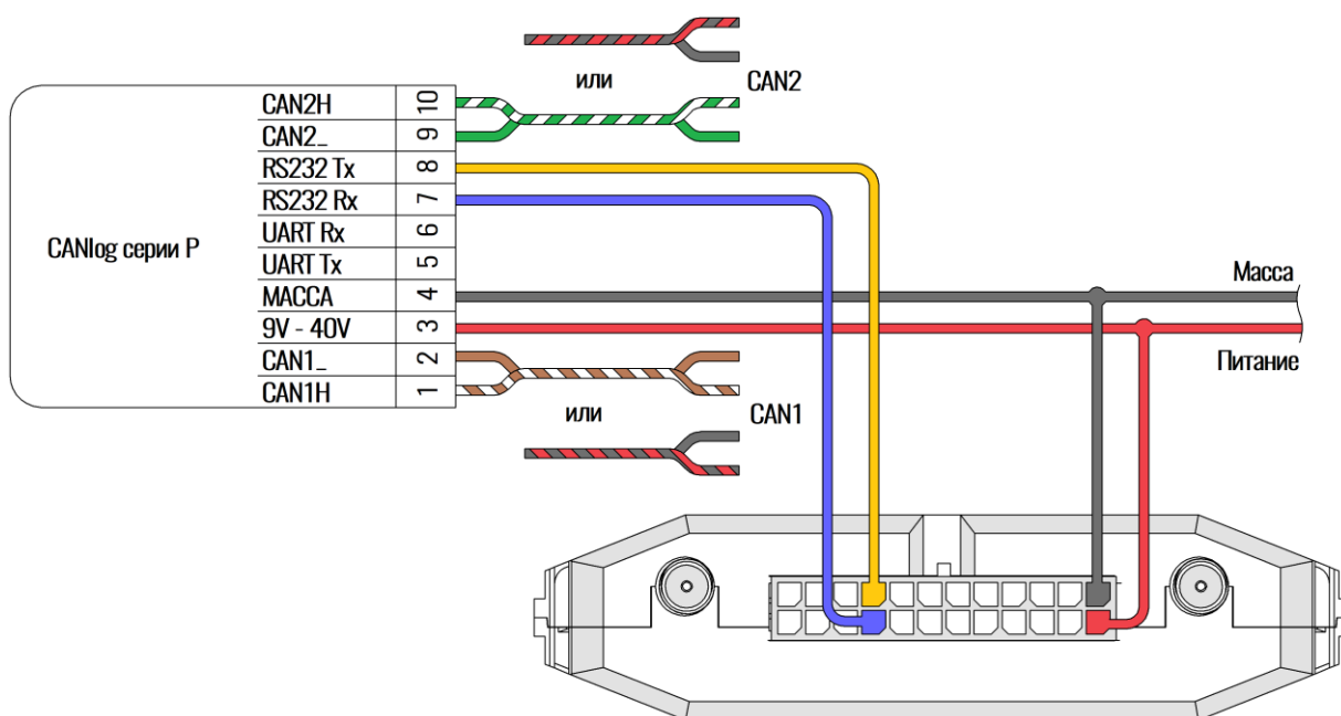
Рисунок 2.23 Подключение CAN-LOG по RS-232
