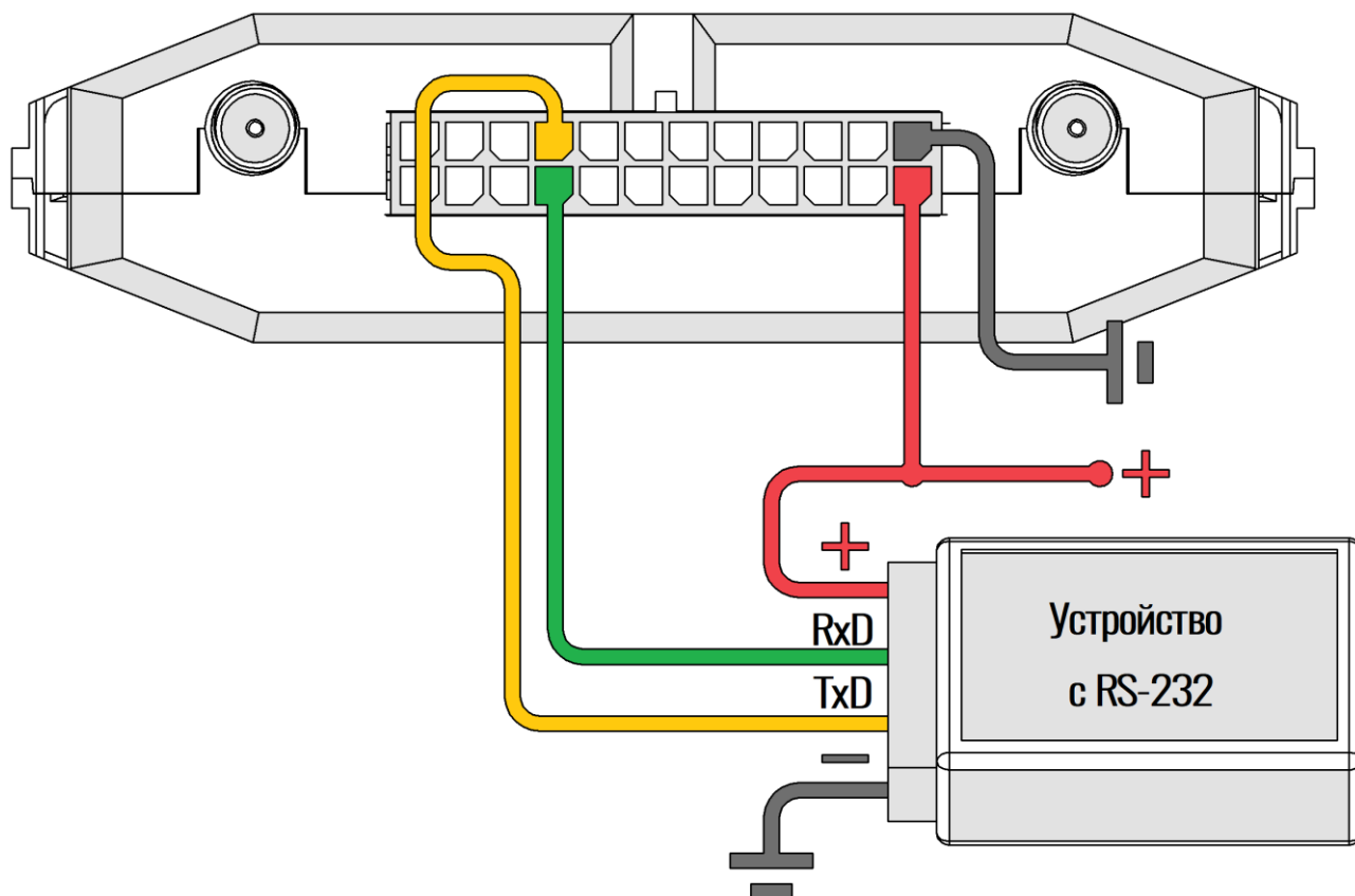
Рисунок 2.21 Подключение по интерфейсу RS-232
