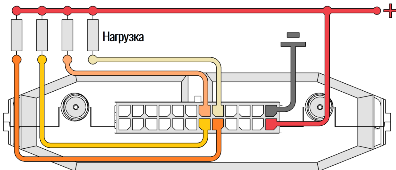
Рисунок 2.15 Подключение маломощной нагрузки
