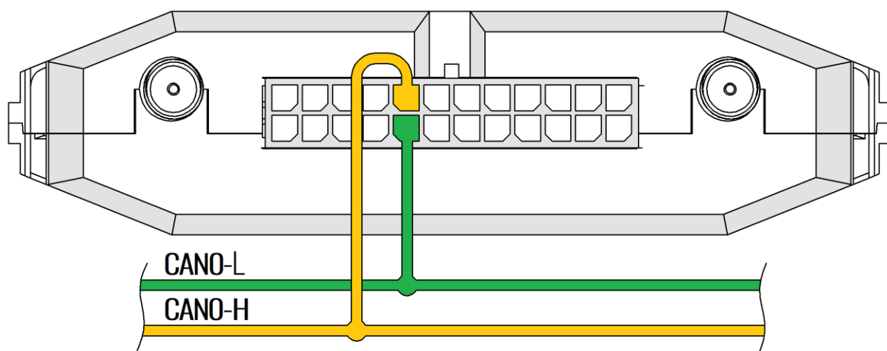
Рисунок 2.20 Подключение к шине CAN
