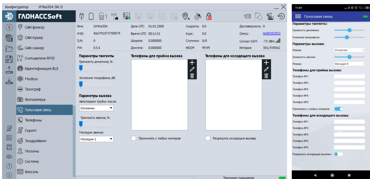
Рисунок 3.43 Вкладка «Голосовая связь»
