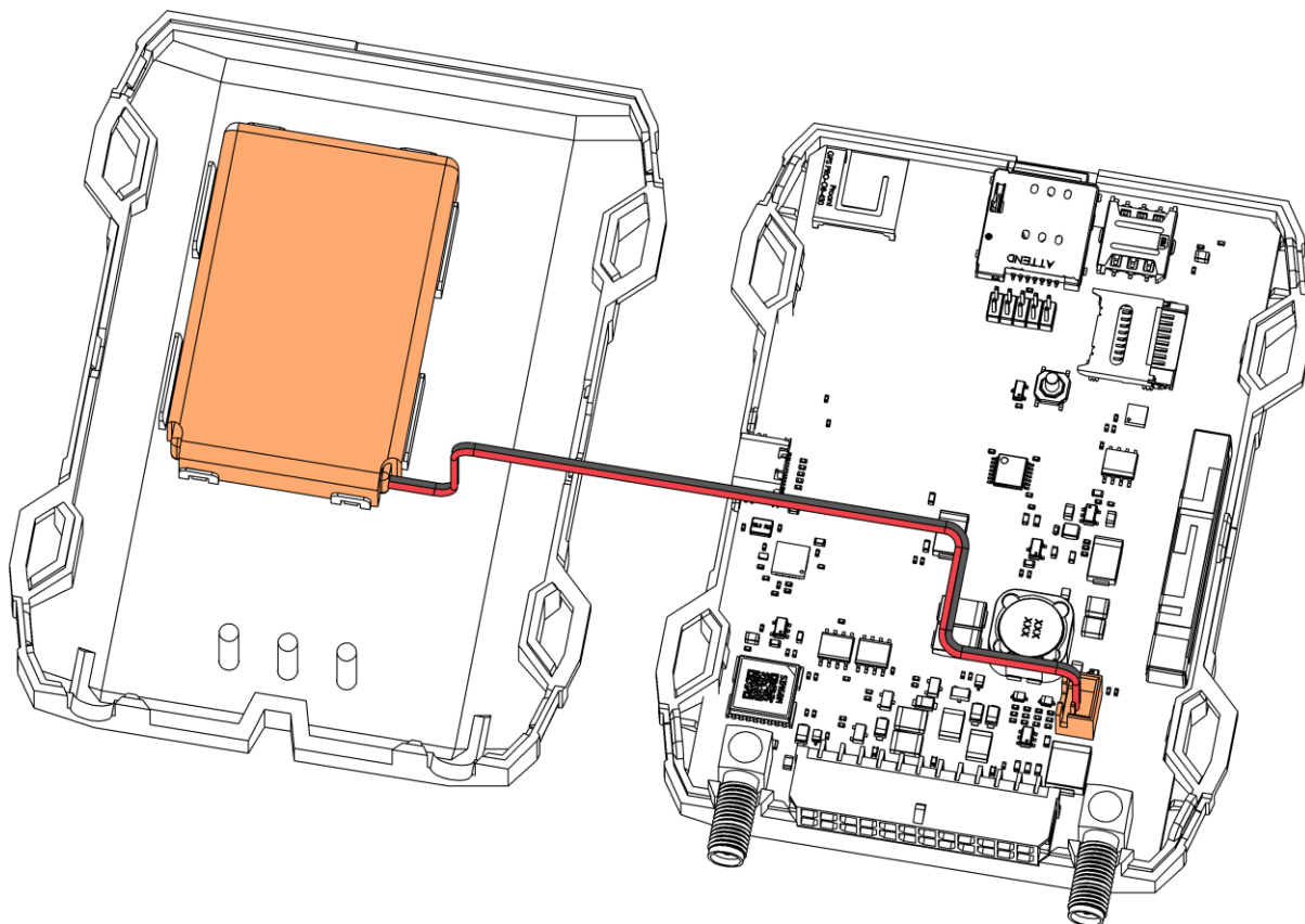
Рисунок 2.5 Установка аккумулятора
