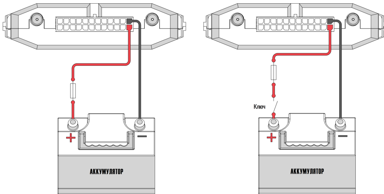
Рисунок 2.7 Подключение питания
