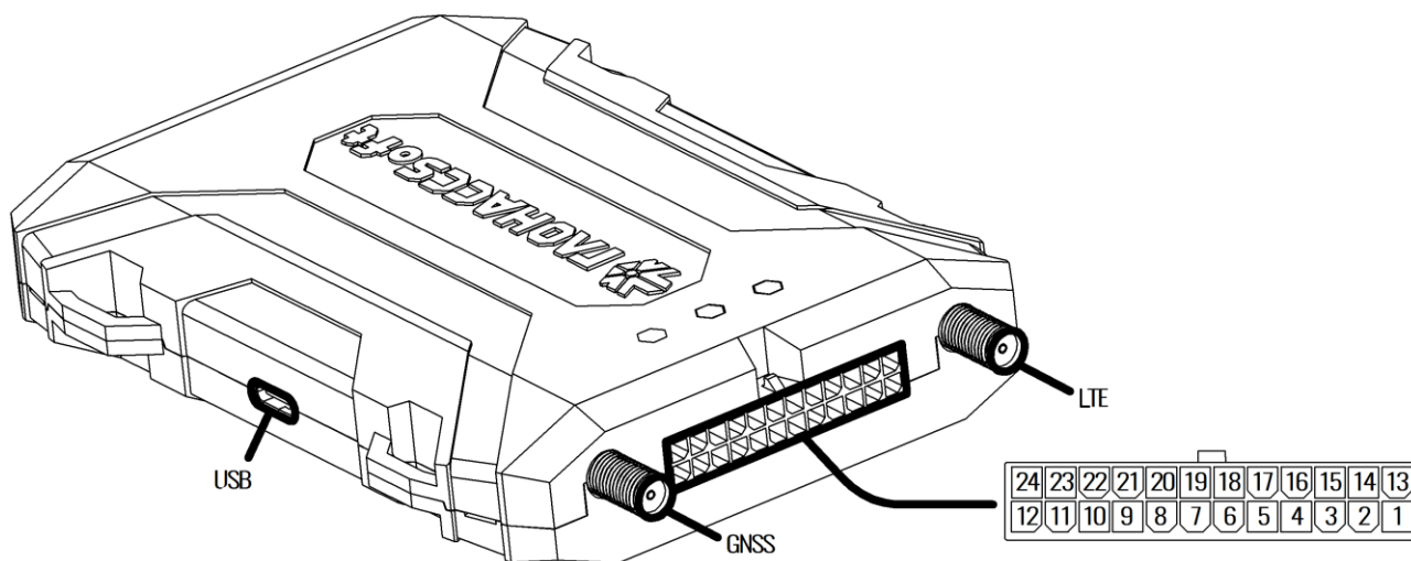
Рисунок 2.2 Нумерация выводов терминала
