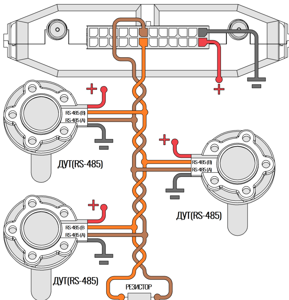
Рисунок 2.17 Подключение ДУТ по интерфейсу RS-485
